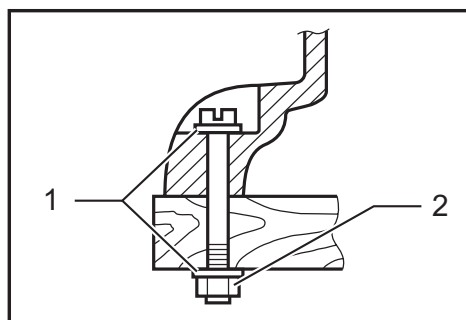
► 1. Arandela normal de 6 mm (1/4") 2. Apretar firmemente el perno y arandela de montaje de 6 mm (1/4")
