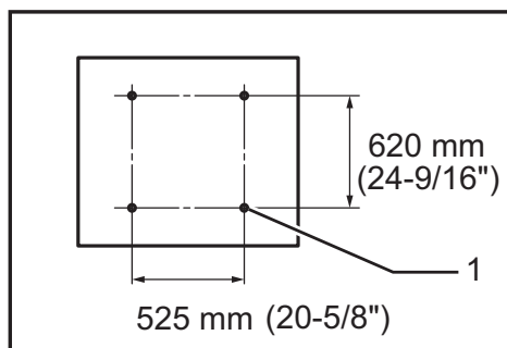
► 1. Diamètre d'orifice 8 mm (5/16")
