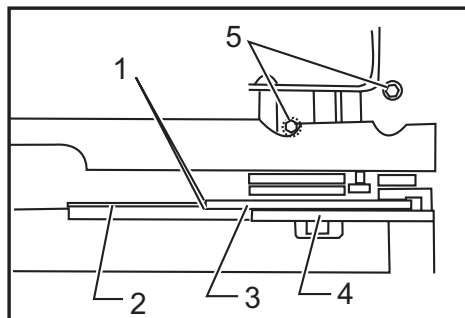
► 1. Ces deux espaces libres doivent être égaux 2. Fer 3. Couteau diviseur/séparateur 4. Plaque de pression 5. Boulons hexagonaux
