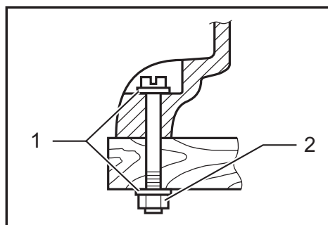
► 1. Rondelle ordinaire de 6 mm (1/4") 2. Boulon et écrou de montage de 6 mm (1/4") – Serrer fermement
