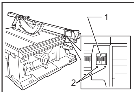
► 1. Guideline 2. Screws
