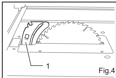
► 1. Couteau diviseur/séparateur en position Couteau diviseur
