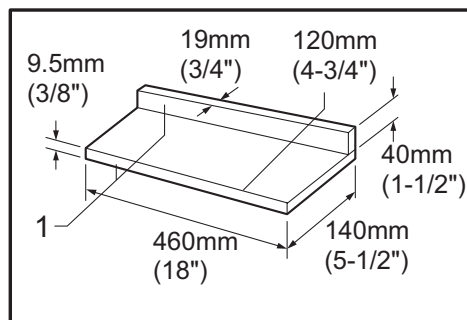
► 1. Cara/borde paralelos
