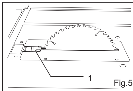
► 1. Couteau diviseur/séparateur en position Dado
