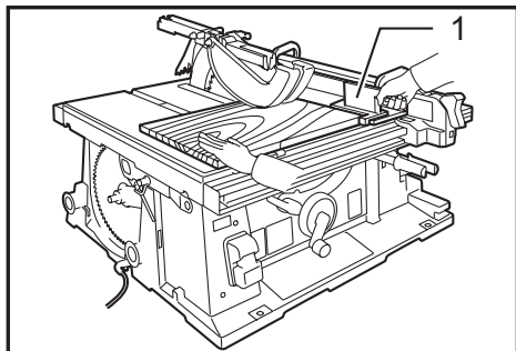
► 1. Bloc-poussoir
