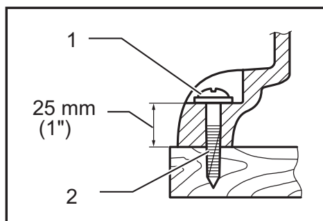
► 1. Rondelle ordinaire de 6 mm (1/4") 2. Vis à bois no 10, longueur min. 40 mm (1-1/2")
