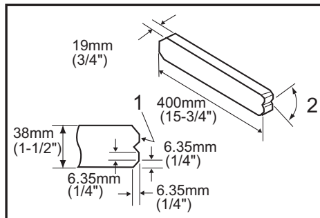
► 1. Extrémité de la pièce 2. Encoche à 45°
