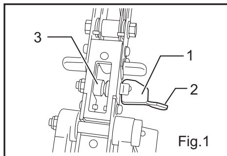
► 1. Levier de verrouillage en position déverrouillée 2. Languette de levier de verrouillage 3. Broche de levier de verrouillage
